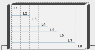
Bočne lajsne LB Bočne lajsne za plakare bez rasvete ŠxVxD: 2,5x226x17,5cm
